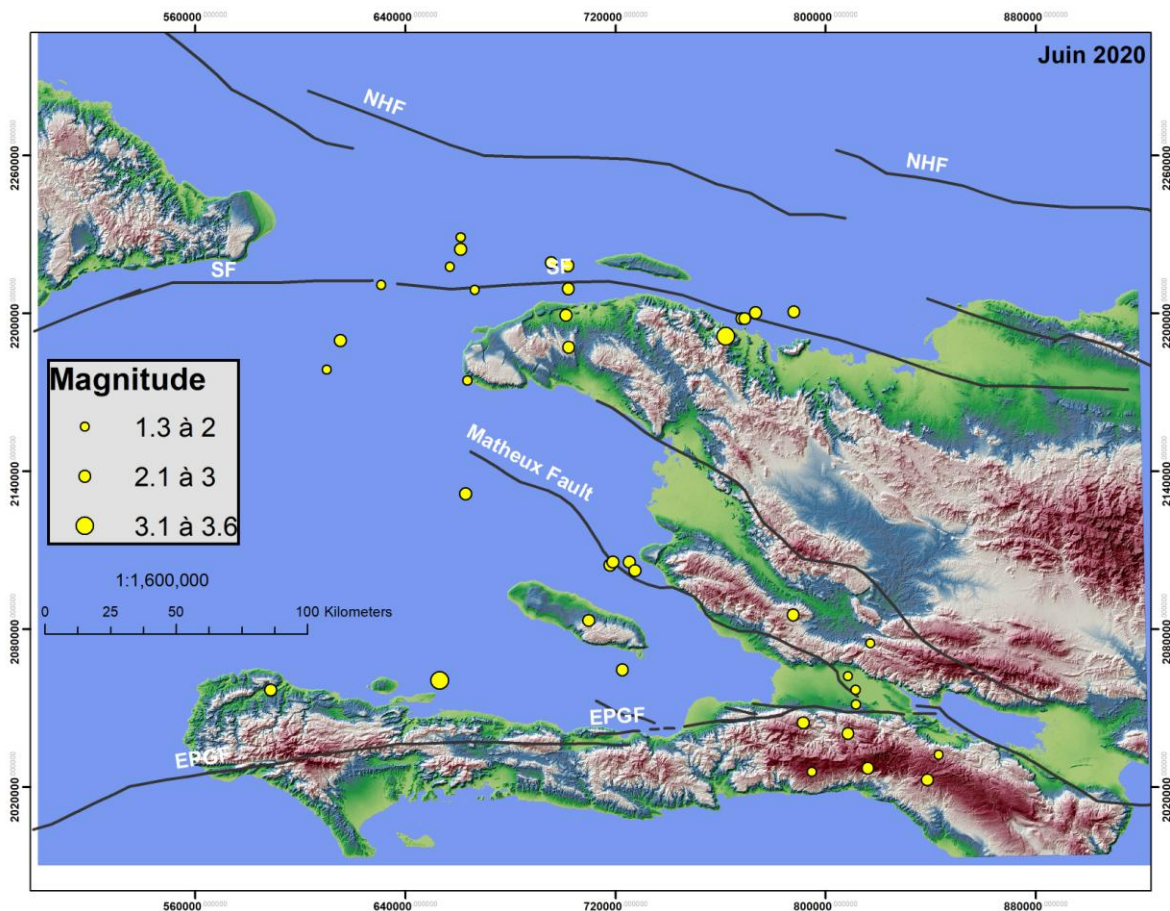
Carte des séismes enregistrés en Haïti au cours du mois de juin 2020
