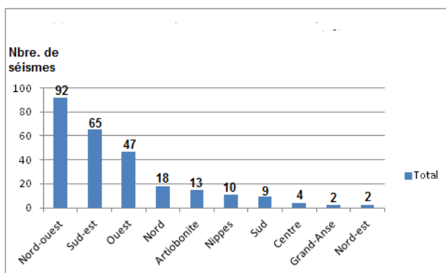
Histogramme des séismes par départements géographiques de janvier à juin 2020
