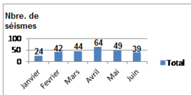
Histogramme des séismes de janvier à juin 2020
